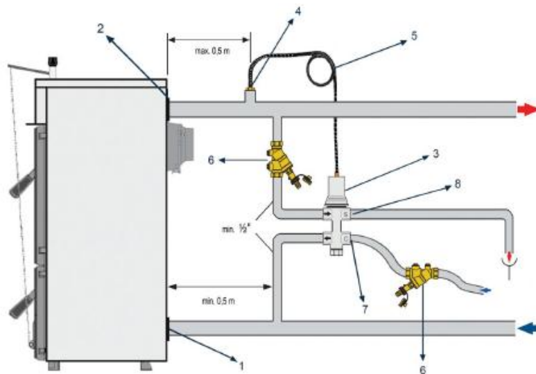
Obrázok 1 Pretlakové bezpečnostné zariadenie
